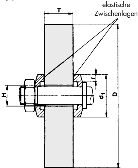
Bild 1: Ringflächenhöhe r von Spannflanschen bei Schleifscheiben H \leq 0,2 D
