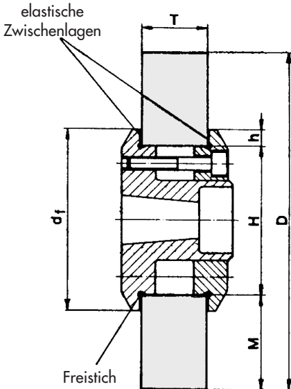
Bild 2: Ringflächenhöhe h von Spannflanschen bei Schleifscheiben H > 0,2 D
